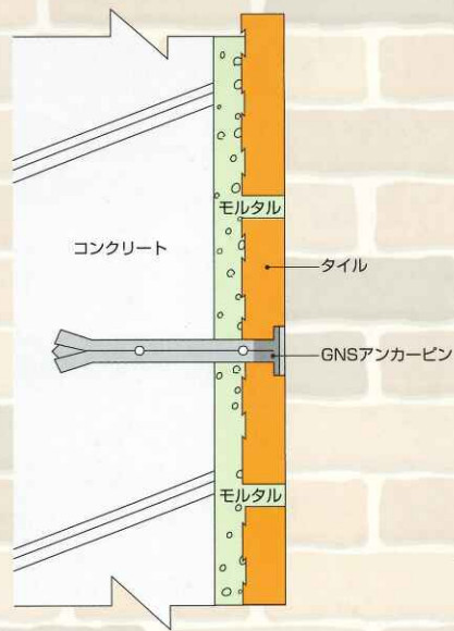
施工断面図
